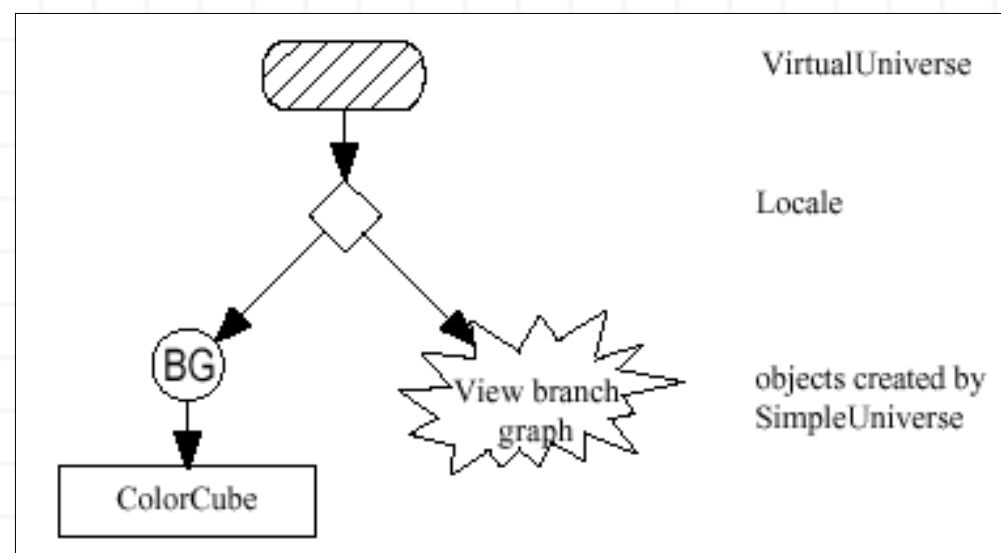
Figura 1-11 Escenario Gráfico del ejemplo HelloJava3Da
