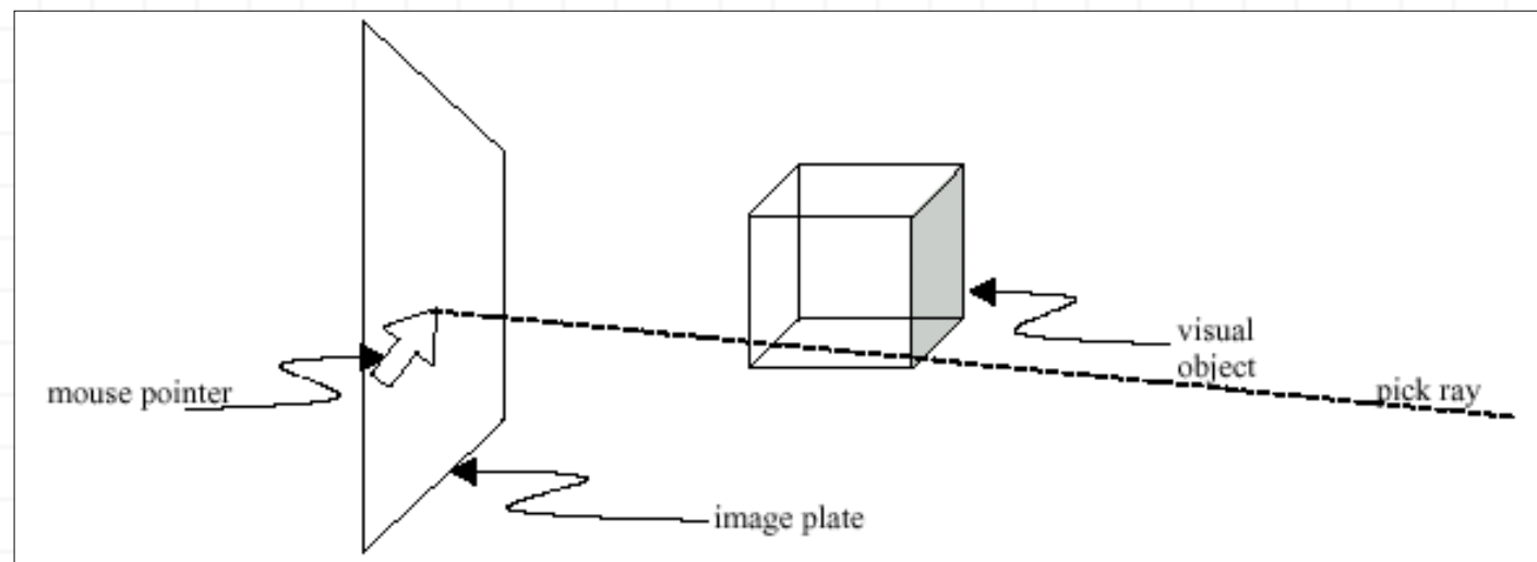
Figura 4-11, Proyección de un PickRay en el Mundo Virtual
