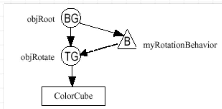
Figura 4-4, Diagrama del Escenario Gráfico de la Rama de Contenido Gráfico de SimpleBehaviorApp.java.
