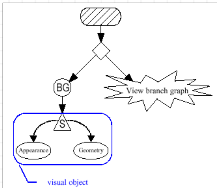
Figura 2-2. Un Objeto Shape3D Define un Objeto Visual en un Escenario Gráfico
