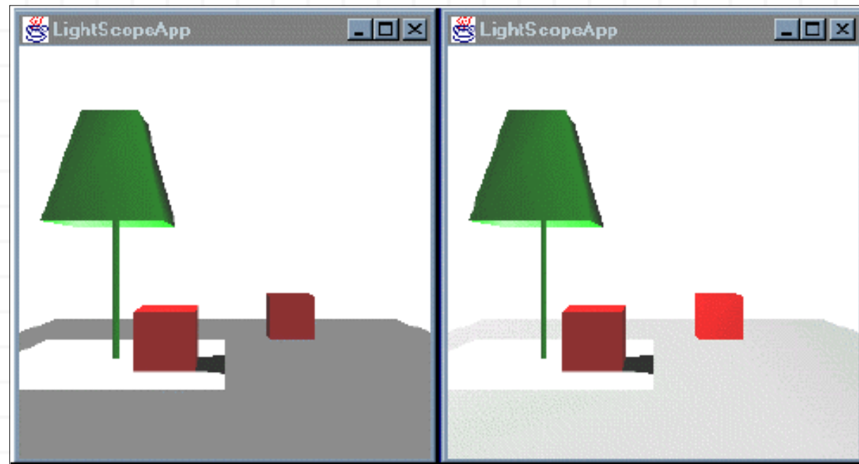
Figura 6-25, Ejemplo de Escena con y sin ámbito de Luz.
