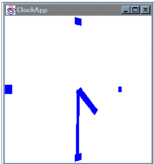
Figura 5-5, Escena renderizada a las 4:30 por el programa de ejemplo ClockApp.
