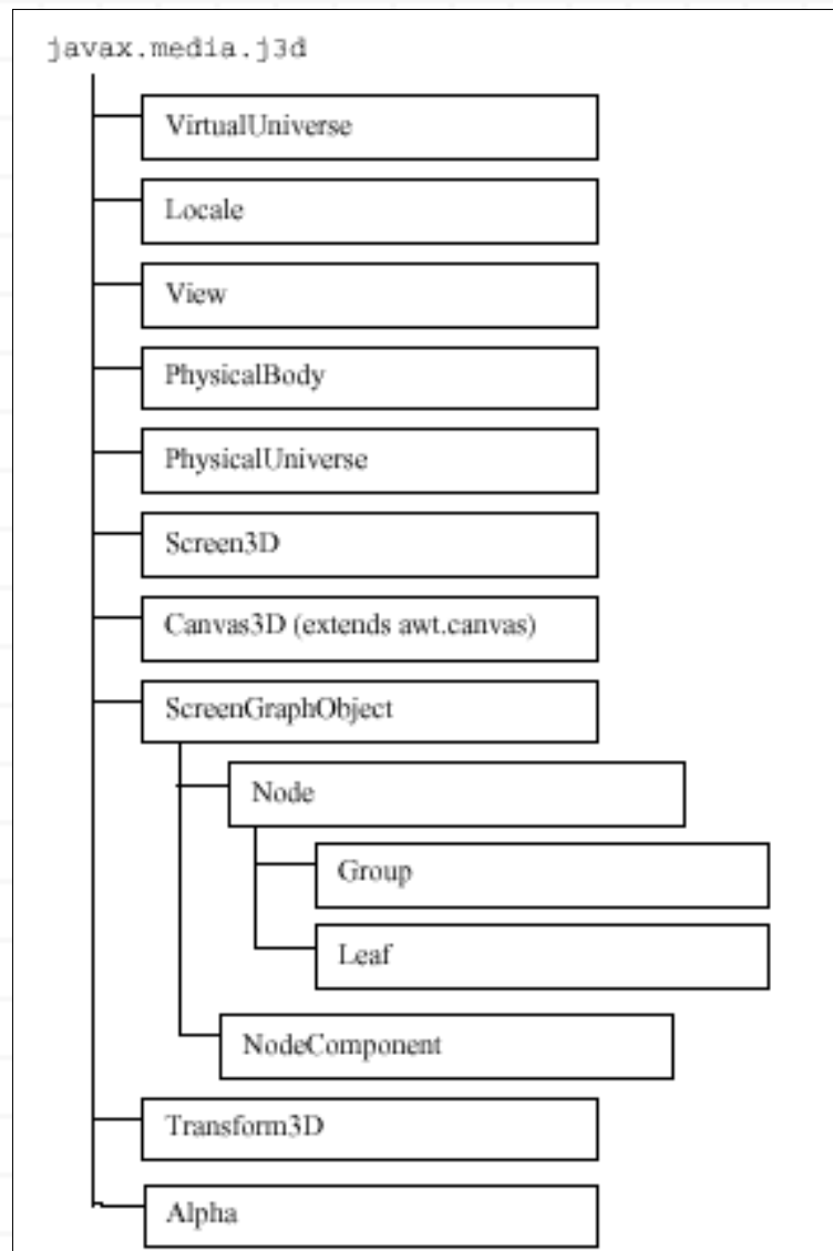
Figura 1-5. Introducción al Árbol de Clases de API Java 3D
