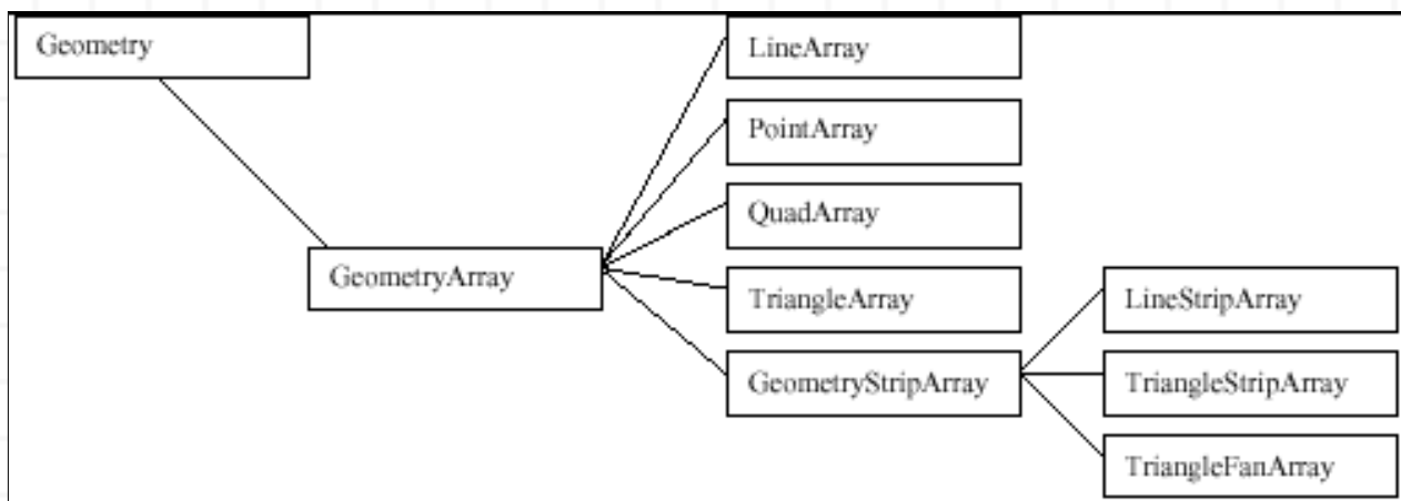
Figura 2-12. Subclases no indexadas de GeometryArray.
