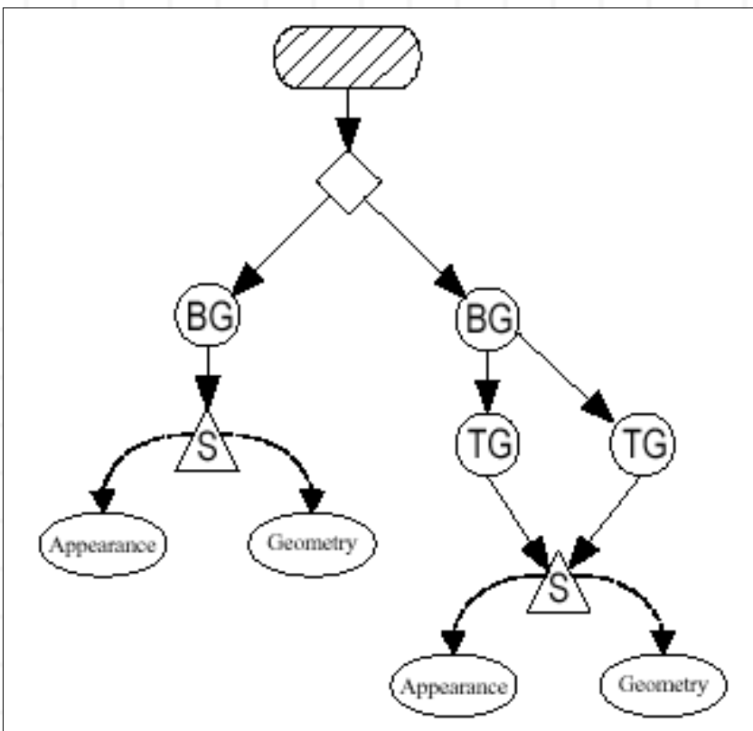
Figura 1-3. Un Escenario Gráfico Ilegal
