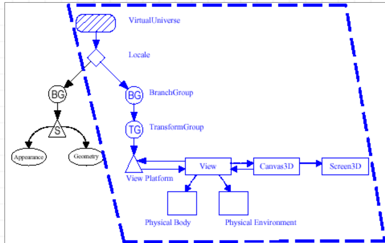
Figura 1-7. La clase SimpleUniverse proporciona un universo virtual mínimo, indicado por la línea punteada azul
