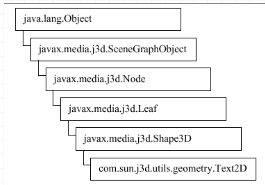
Figura 3-7, El Árbol de Clases de Text2D
