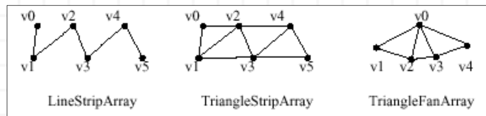
Figura 2-14. Subclases de GeometryStripArray.
