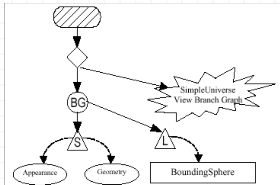
Figura 6-6, Diagrama de Escenario Gráfico del Fragmento de Código 6-1
