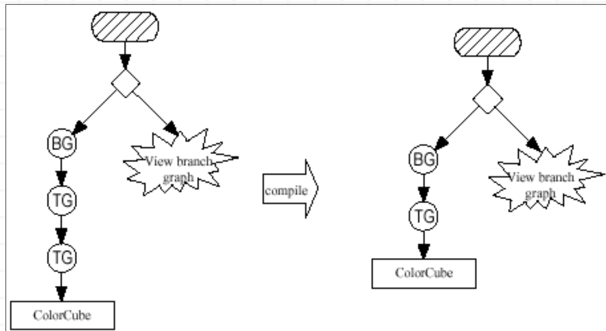
Figura 1-16 Ejemplo Conceptual del Resultado de Compilar un Escenario Gráfico
