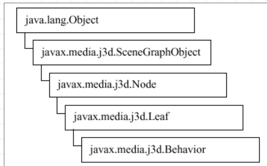
Figura 4-6, Árbol de Clases de Behavior
