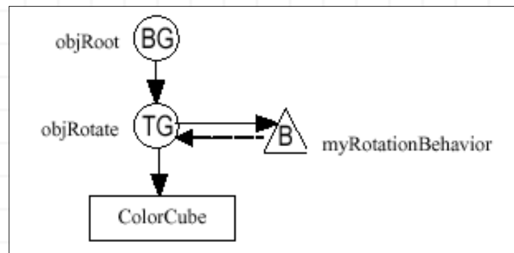
Figura 4-5, Una alternativa a la situación del escenario gráfico para el objeto Behavior en SimpleBehaviorApp.
