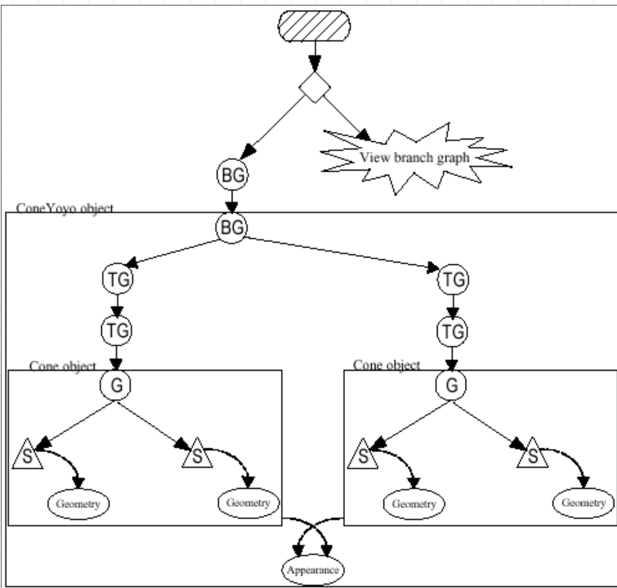
Figura 2-6. Escenario Gráfico de la Aplicación ConeYoyo
