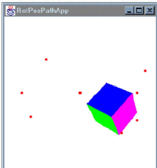
Figura 5-13, una escena renderizada por RotPosPathApp mostrando la interpolación de la Rotación y Posición de un ColorCube. Los puntos rojos muestran los nudos de la aplicación de ejemplo.
