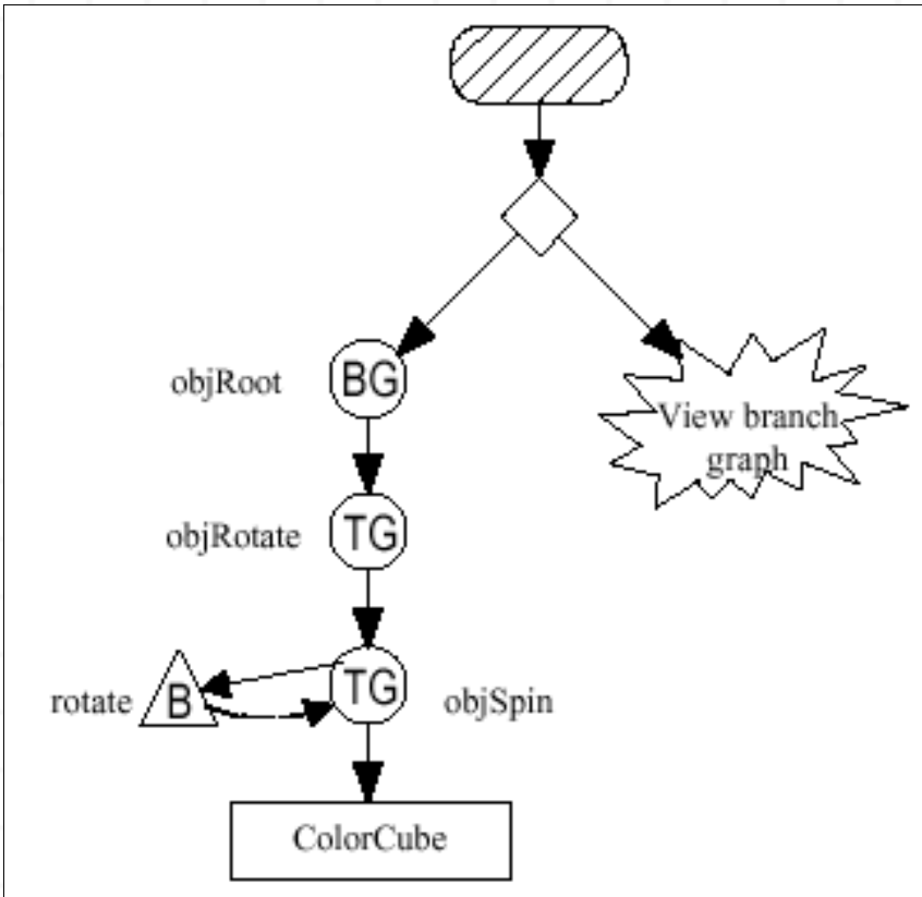
Figura 1-20 Escenario Gráfico del Ejemplo HelloJava3Dd.
