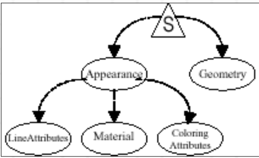
Figura 2-19, un Paquete de Apariencia
