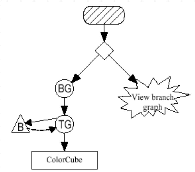
Figura 1-18 Escenario Gráfico del Ejemplo HelloJava3Dc.
