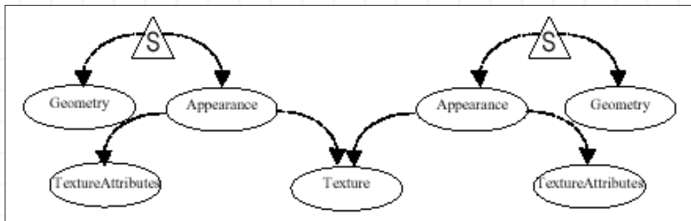
Figura 7-16. Dos objetos visuales compartiendo la misma Textura Personalizada por Componentes TextureAttributes.
