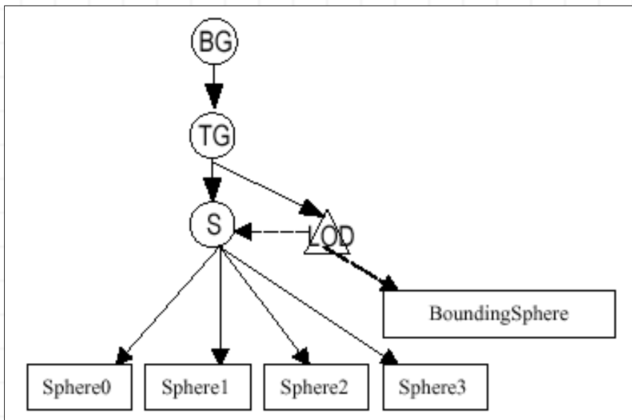
Figura 5-18, Diagrama Parcial del Escenario Gráfico del Programa DistanceLODApp.
