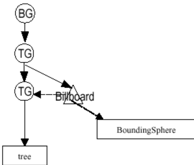
Figura 5-15, Diagrama del Escenario Gráfico que Usa un Objeto Billboard Creado en el Fragmento de Código 5-3.
