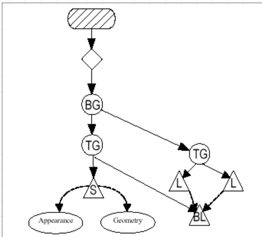
Figura 6-23, Mover un Objeto Light Independientemente de su Influencia usando un BoundingLeaf.
