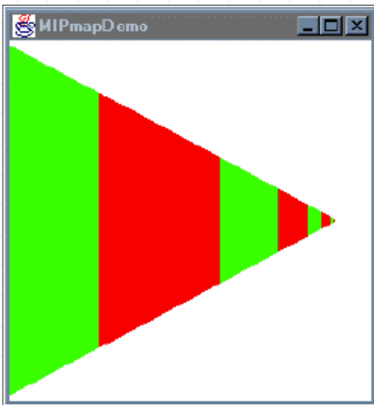
Figura 7-20, La imagen Generada por un Plano texturado con una Textura MipMap multi-color.
