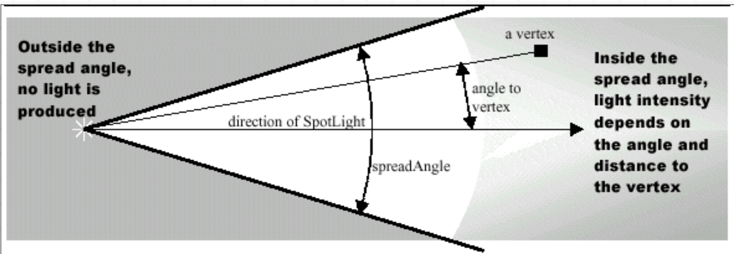
Figura 6-14, La intensidad de Luz varía con la Distancia y la Orientación desde una fuente PointLight.
