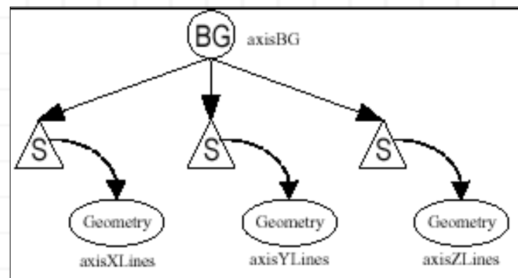
Figura 2-11, La clase Axis de AxisApp.java crea este Escenario Gráfico.
