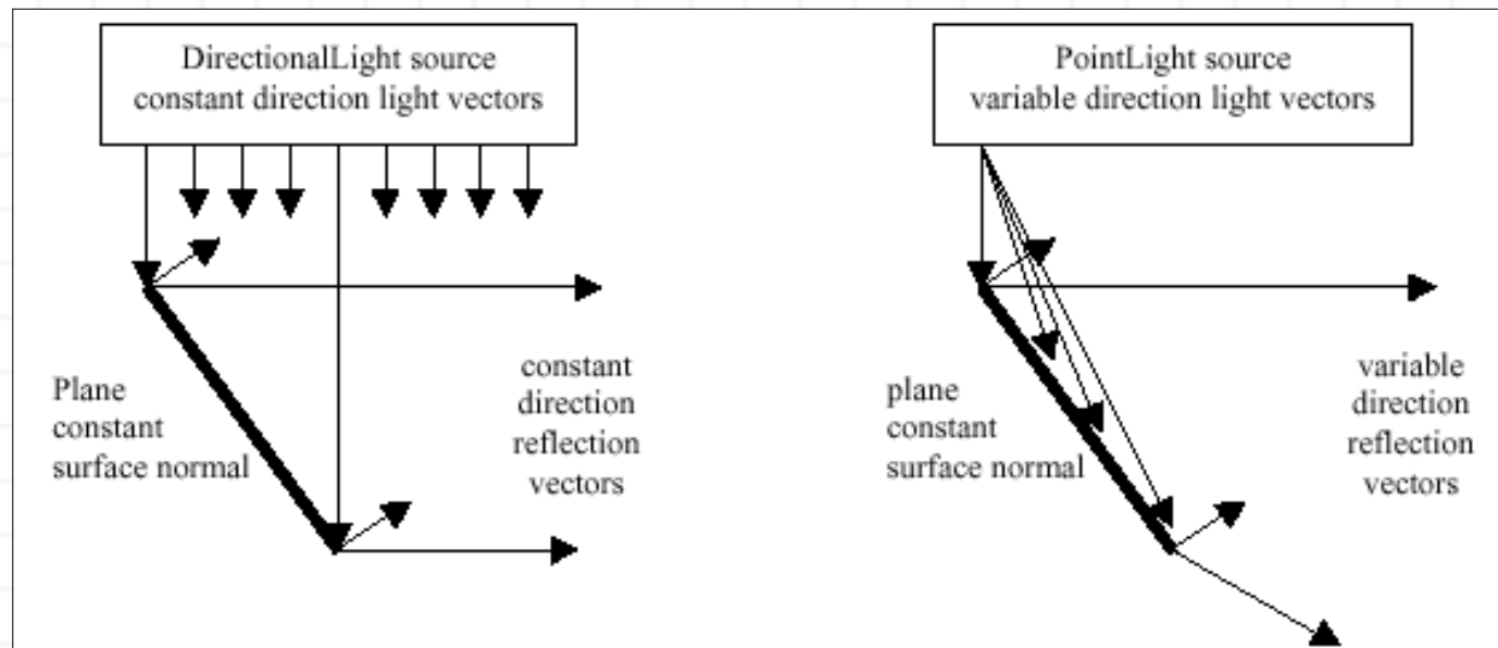
Figura 6-17, Geometría de Planos Iluminados con Fuentes de Luces Direccionales y de Punto
