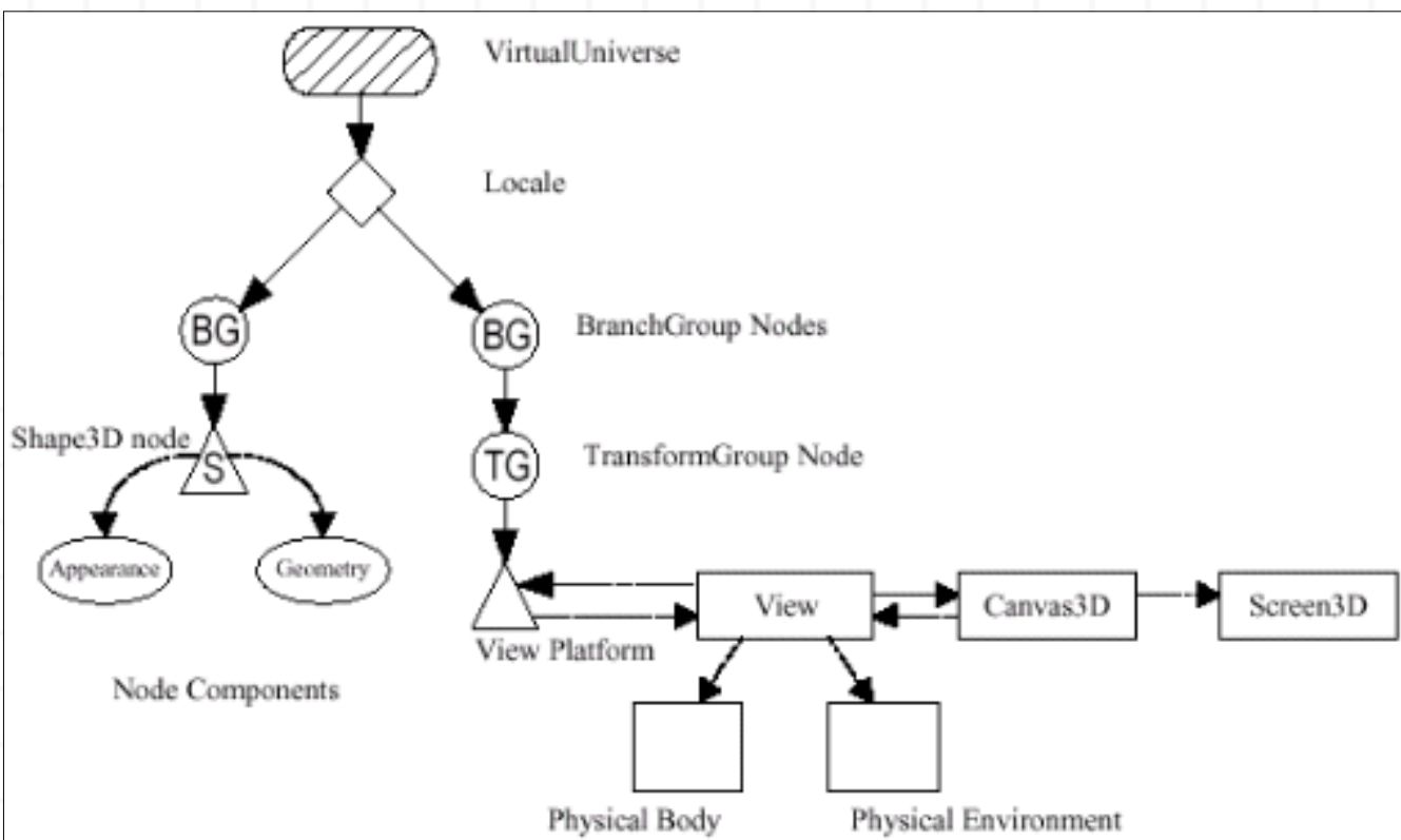
Figura 1-2. Primer Ejemplo de Escenario Gráfico
