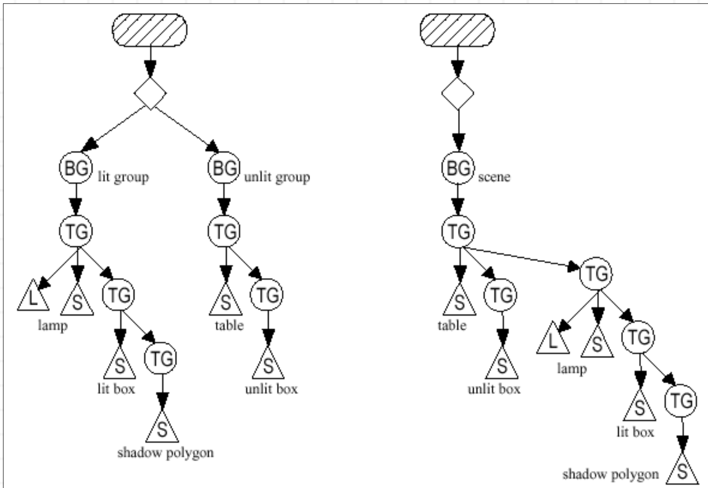
Figura 6-24. Dos posibles Escenarios Gráficos para el Ejemplo de Ambito de Luz.
