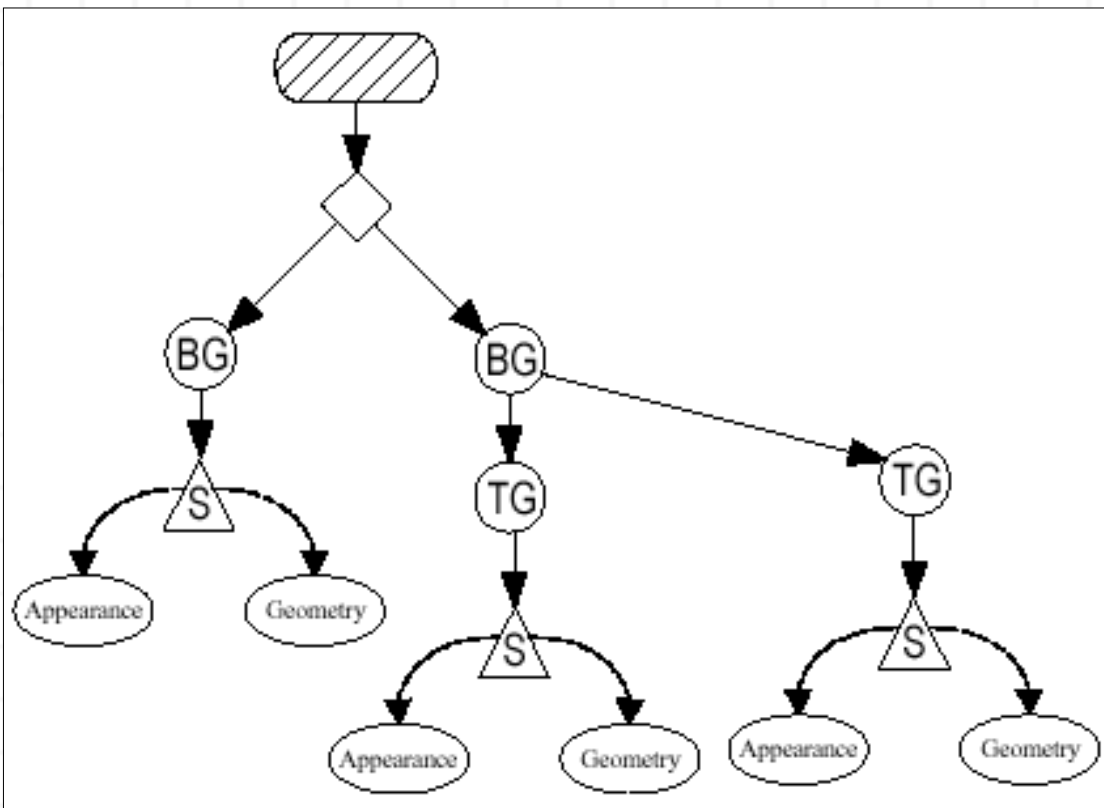
Figura 1-4. Posible solución al escenario gráfico ilegal de la Figura 1-3
