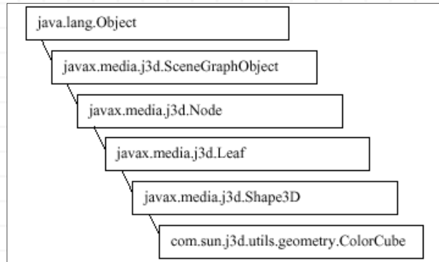
Figura 2-5. Árbol de Clases de la Clases de utilidad ColorCube
