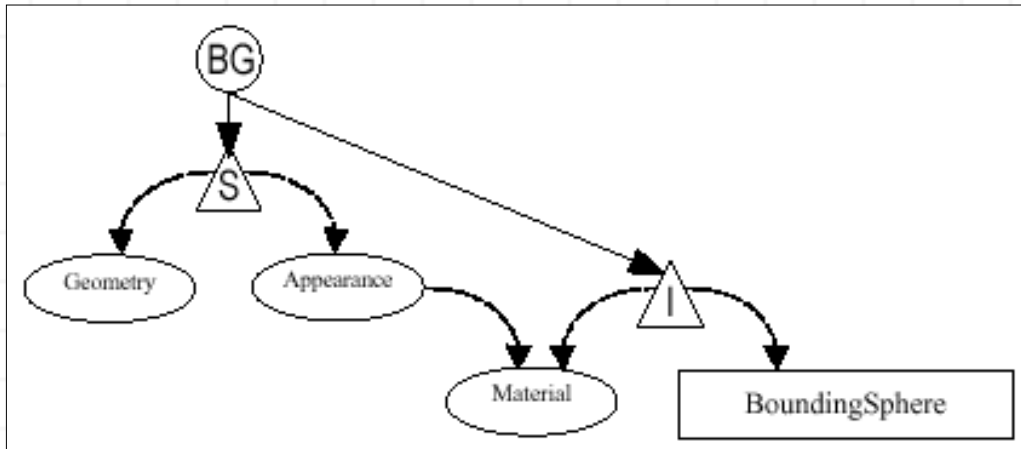
Figura 5-10, Escenario gráfico parcial de un objeto ColorInterpolator y su objeto fuerza Material NodeComponent.
