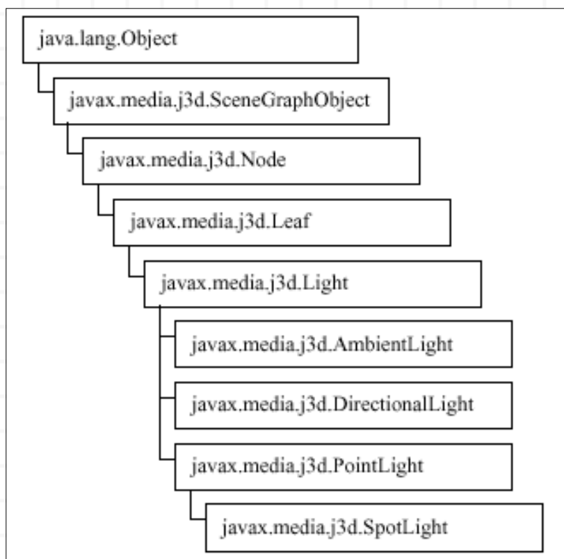
Figura 6-11, El Árbol de Clases del API Java 3D con las clases Light
