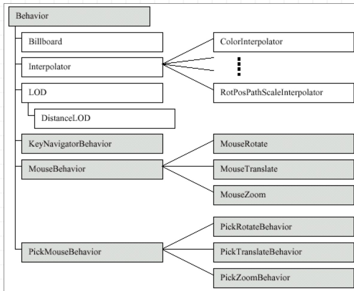
Figura 4-1, Árbol de Subclases de Behavior
