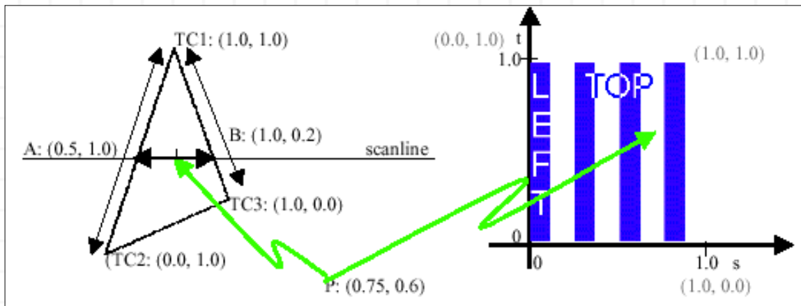
Figura 7-7, Imagen del Mapeo de Textura
