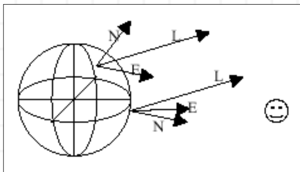
Figura 6-12, El Vector de Luz es Constante para Fuentes DirectionalLight.
