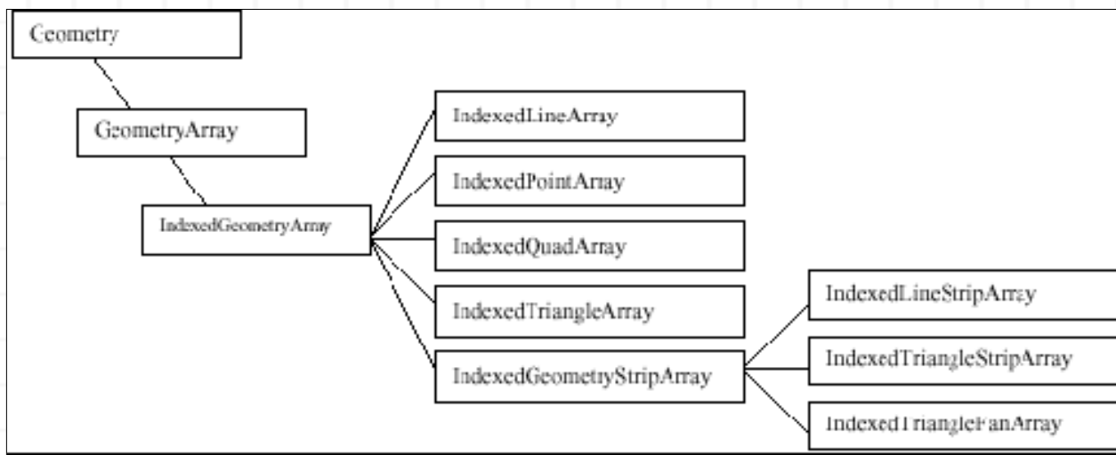
Figura 2-18, Subclases de IndexedGeometryArray
