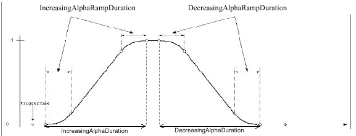
Figura 5-6, Suavizar la forma de onda producida por Alpha 9
