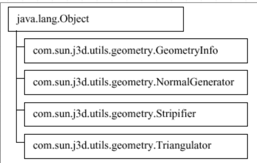
Figura 3-4, Árbol de clases de GeometryInfo y clases relacionadas
