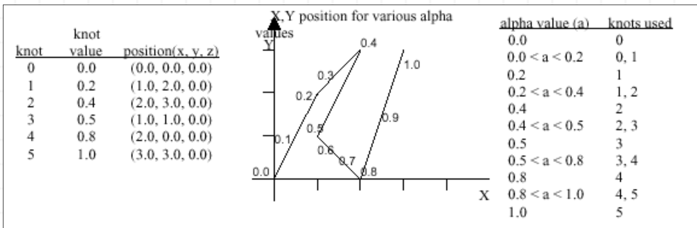
Figura 5-11, la relación entre Nudos y Valores Alpha para un ejemplo de posición 2D.
