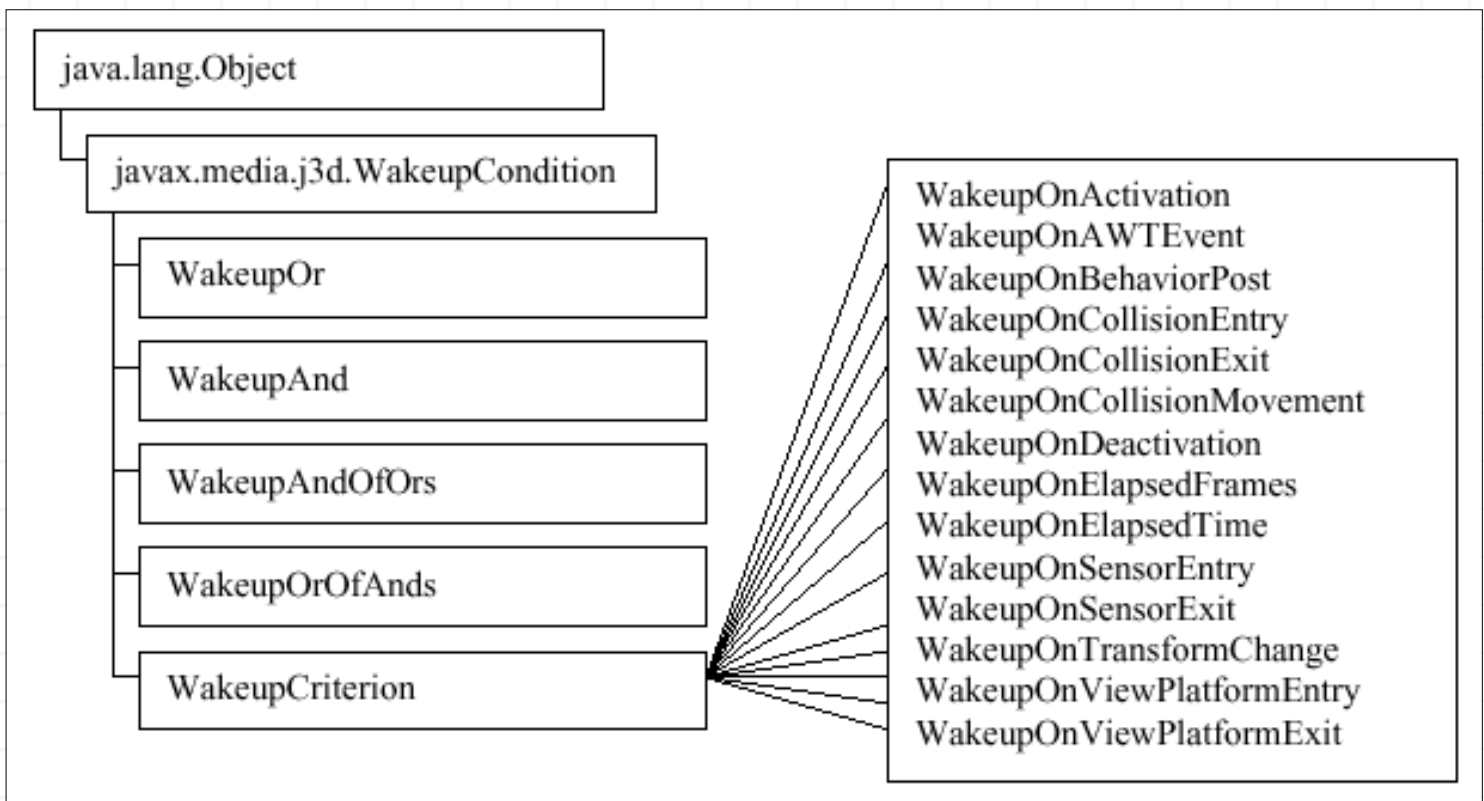
Figura 4-7, el Árbol de Clases para WakeupCondition y clases relacionadas.
