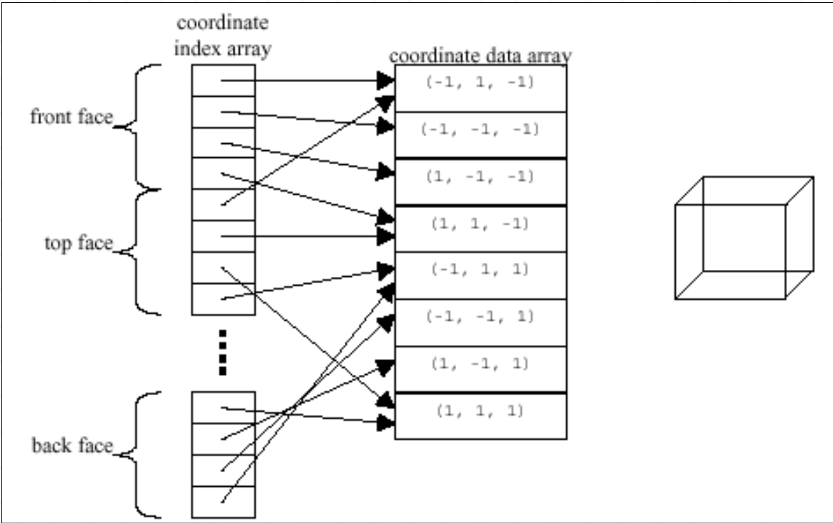
Figura 2-17, Arrays de Índices y de Datos para un Cubo
