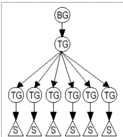
Figura 4-12, Diagrama del Escenario Gráfico para un Cubo Compuesto por objetos Shape3D planos.
