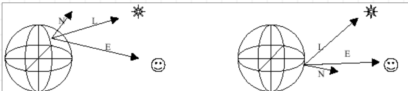
Figura 6-1, Vectores de Luz, Superficie Normal y Ojo del espectador usados para vértices sombreados.
