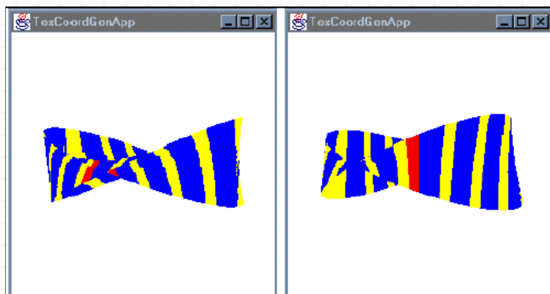
Figura 7-17, Comparar los modos de Generación del objeto TexCoordGeneration.
