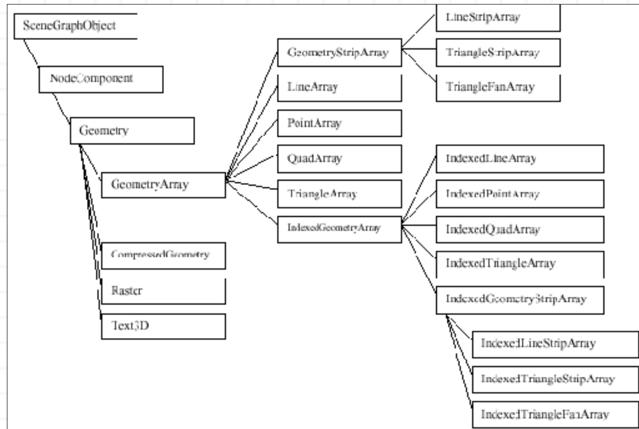
Figura 2-10. Árbol de clases de Geometry.
