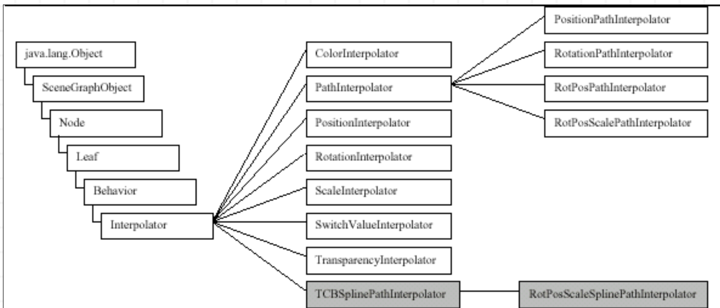
Figura 5-8, Árbol de clases de la clase Interpolator.
