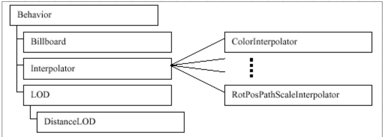
Figura 5-1, Algunas Clases Usadas en Animaciones Java 3D
