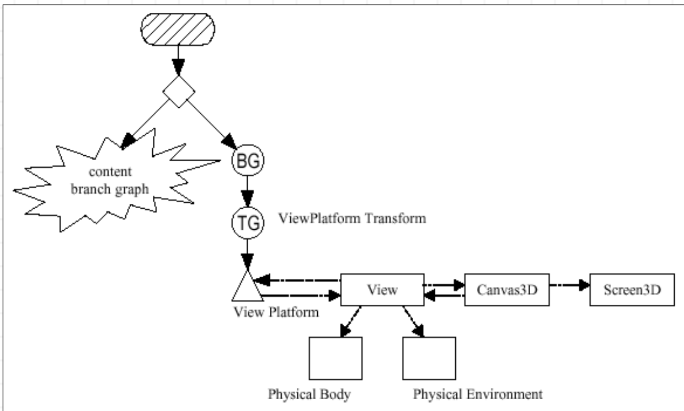
Figura 4-8, la Rama Gráfica Básica mostrando la Transformación de la Vista de la Plataforma
