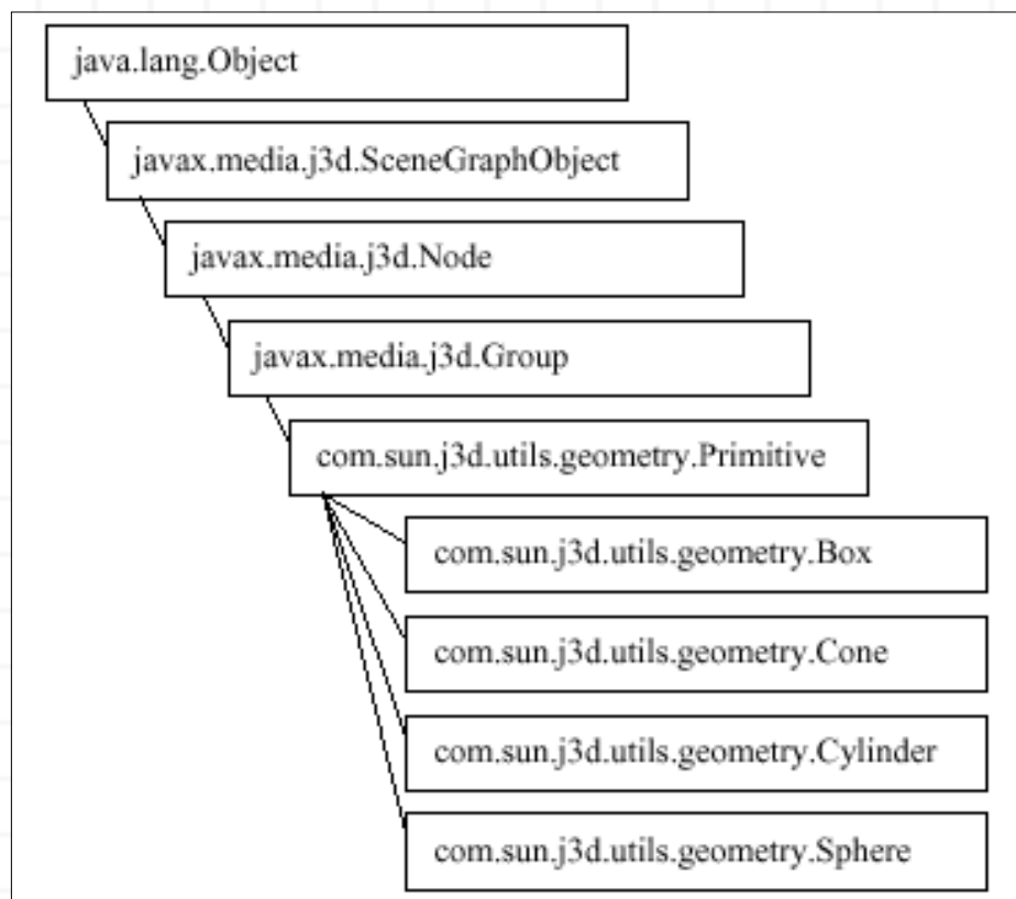
Figura 2-4. Árbol de Clases de las Clases Geométricas Primitivas
