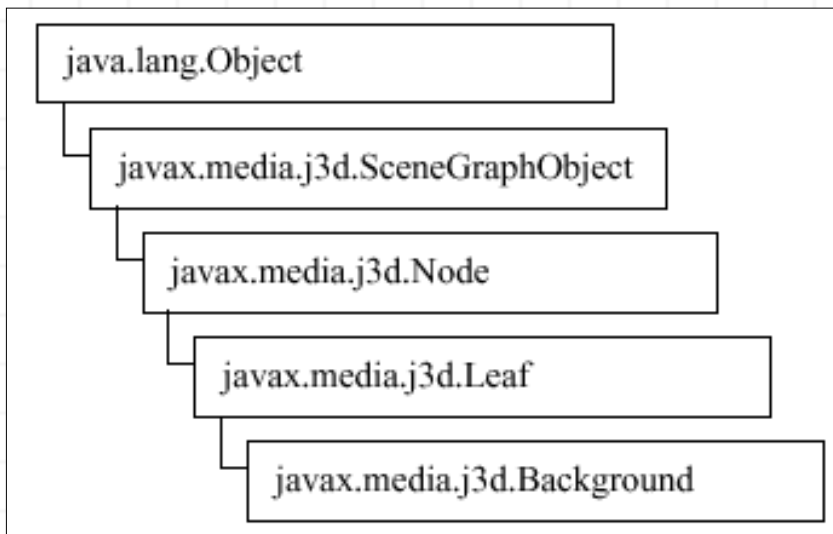
Figura 3-13, Árbol de Clases de Background
