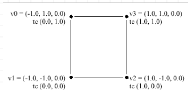
Figure 7-5. La orientación de las Coordenadas de Textura en el Espacio de una Imagen de Textura.
