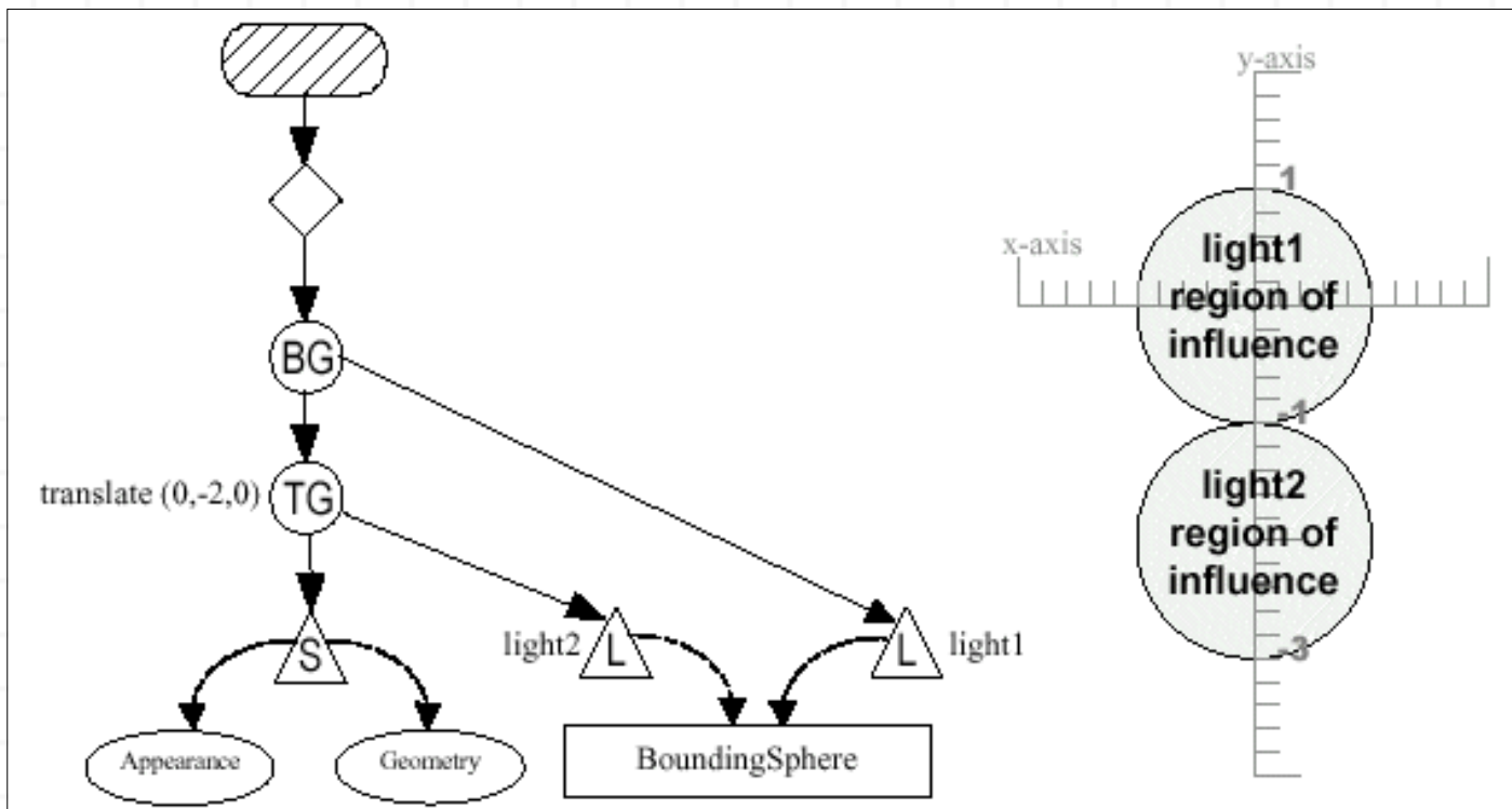
Figura 6-10, un BoundingSphere Afectado por un Transformation
