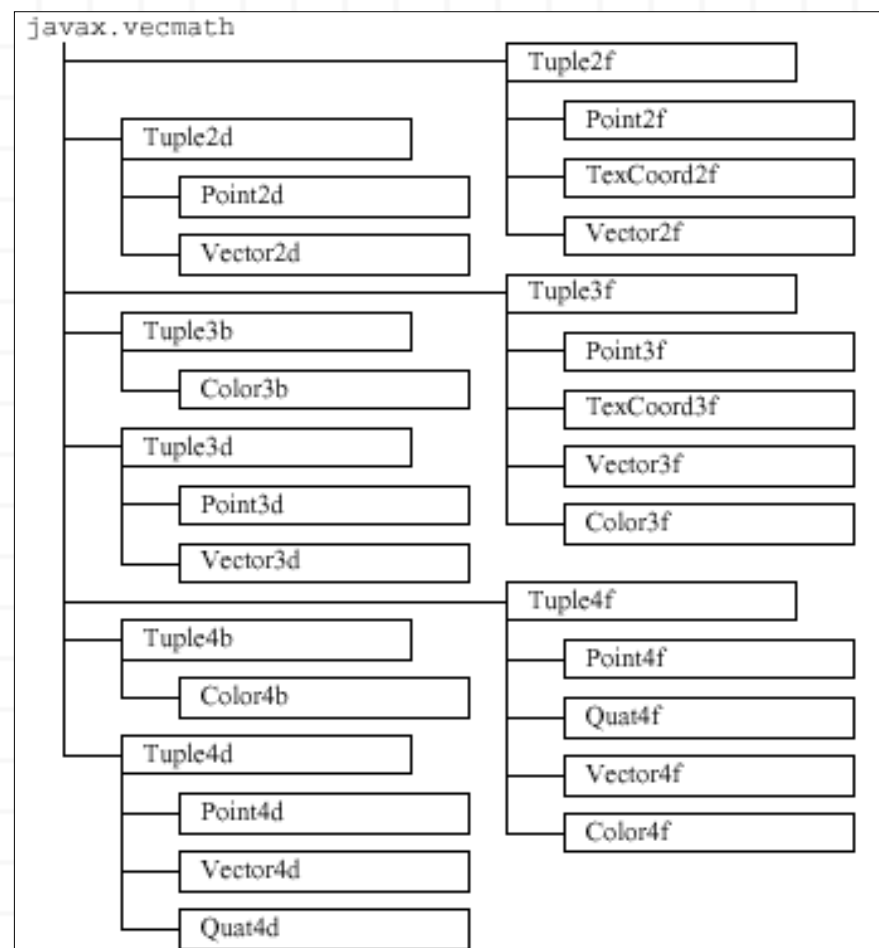
Figura 2-9. Árbol de clases del paquete de clases matemáticas.
