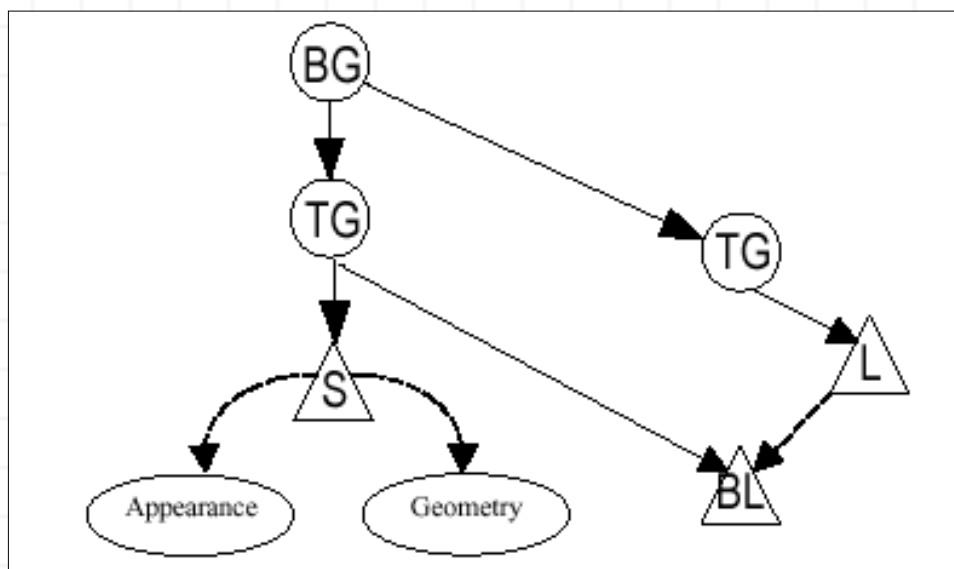
Figura 3-14, un BoundingLeaf se mueve con un objeto visual independientemente de la fuente de luz
