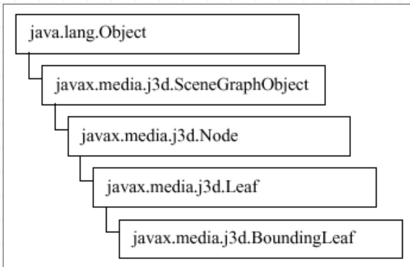
Figura 3-15, Árbol de Clases de la clase BoundingLeaf
