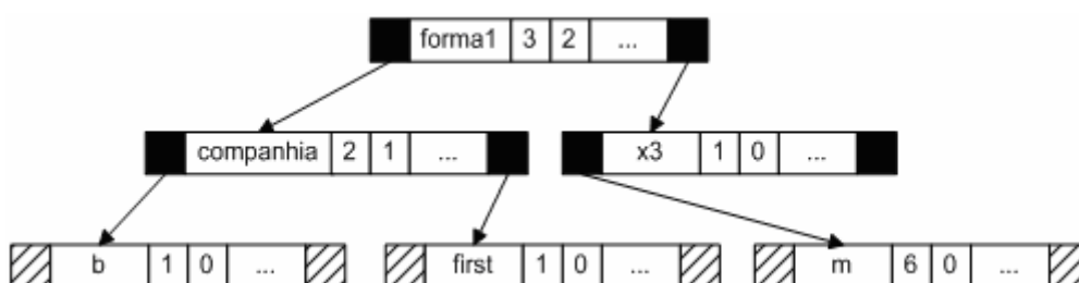
Figura 4-8. Árbol binario equilibrado.
