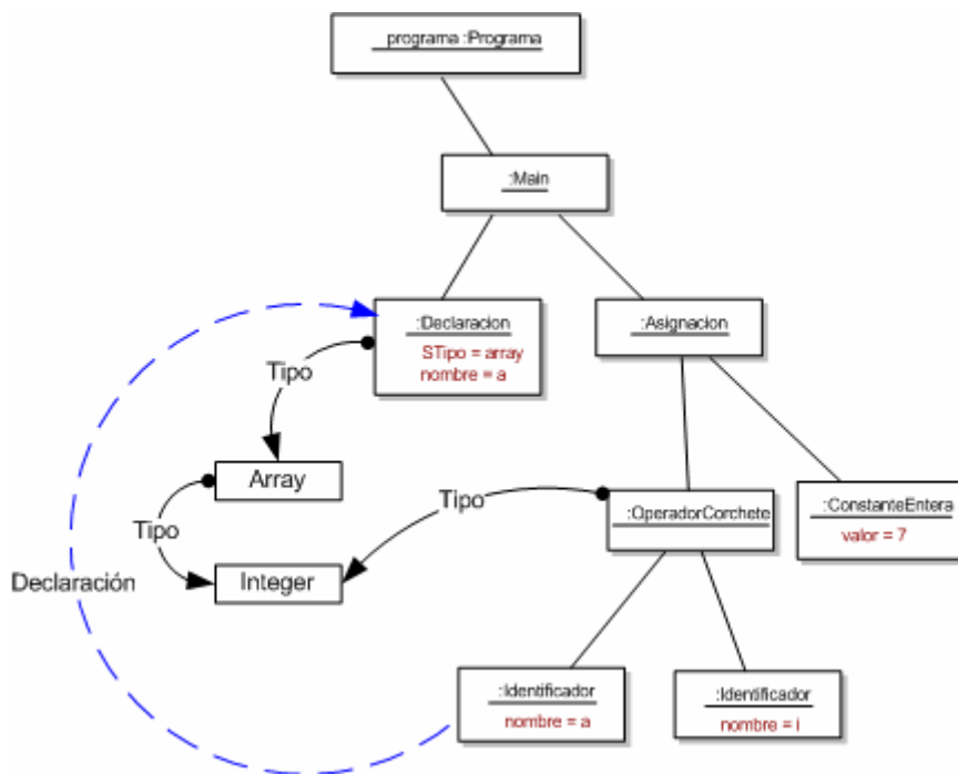
Figura 4-52. Declaración de Arrays
