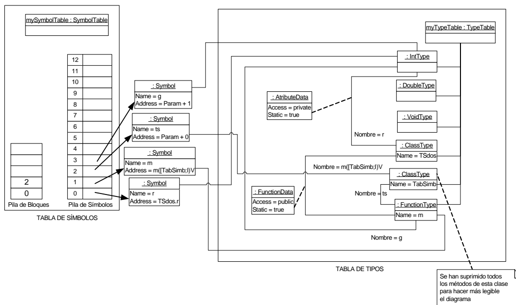
Figura 4-37. Situación de la Tabla de Símbolos después de compilada la línea 11
