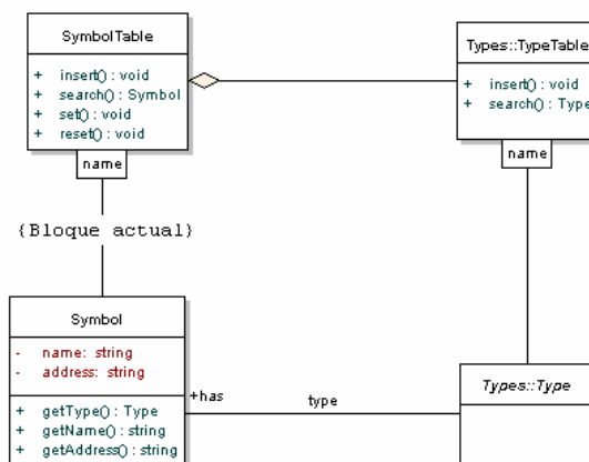
Figura 4-43. Estructura de clases de la TS
