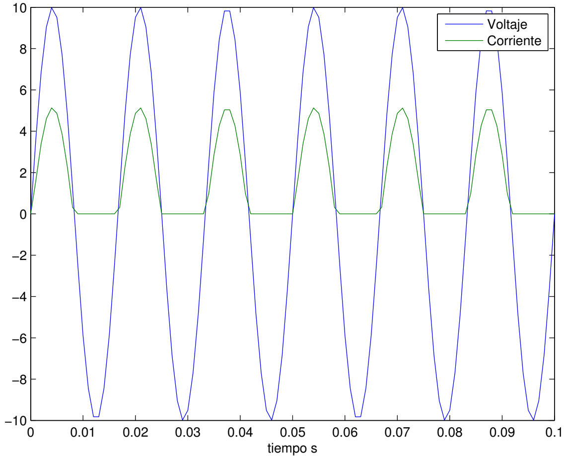
Solución de un circuito con Diodo
