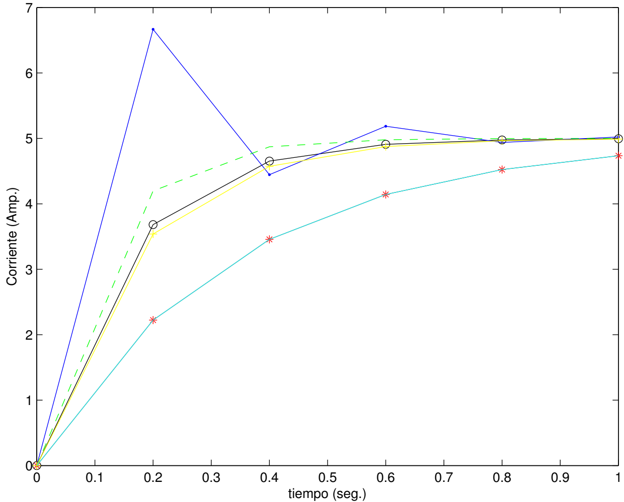
Solucion Circuito RL
