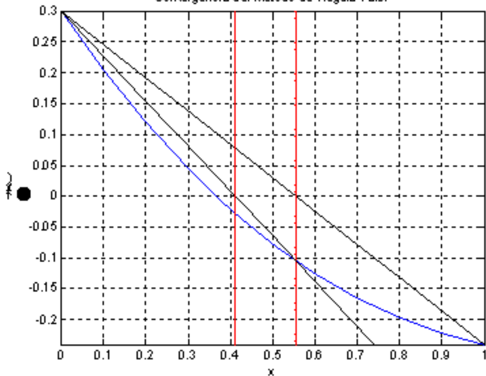
Convergencia del Metodo de Regula Falsi
