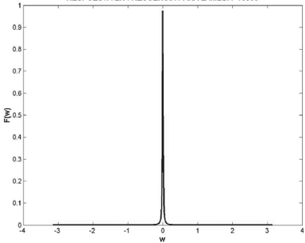
RESPUESTA EN FRECUENCIA PARA LAMBDA=10000
