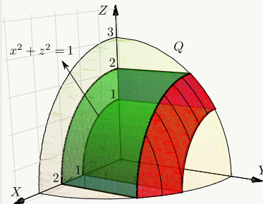
Figura 6.4. Sólido Q
