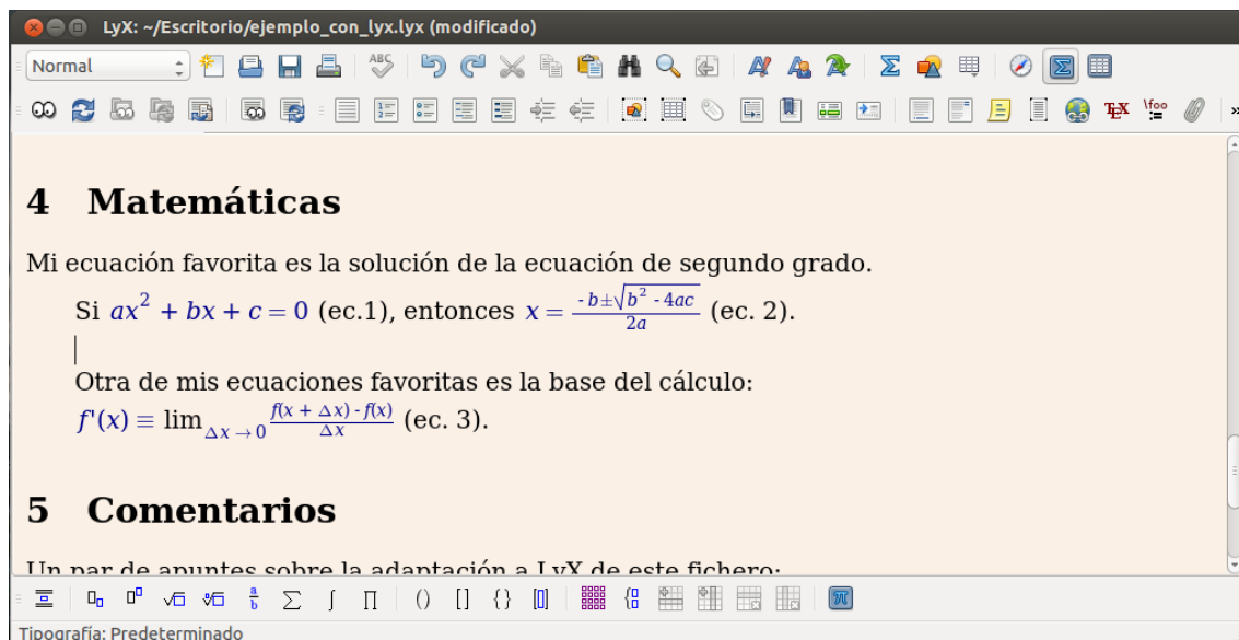
Figura C.4. Editor LyX
