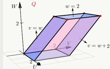
Figura 6.3. Un paralelepípedo
